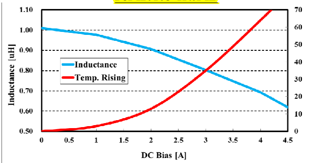
PSM2016S-1R0ML
