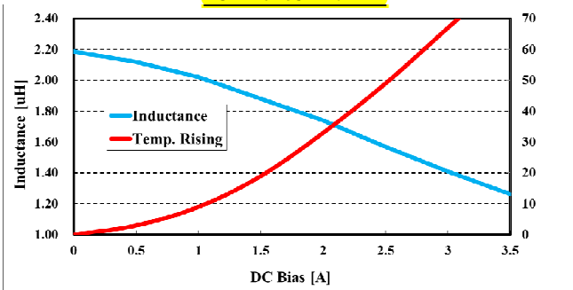
PSM2016S-2R2ML
